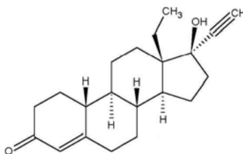
Levonorgestrel
